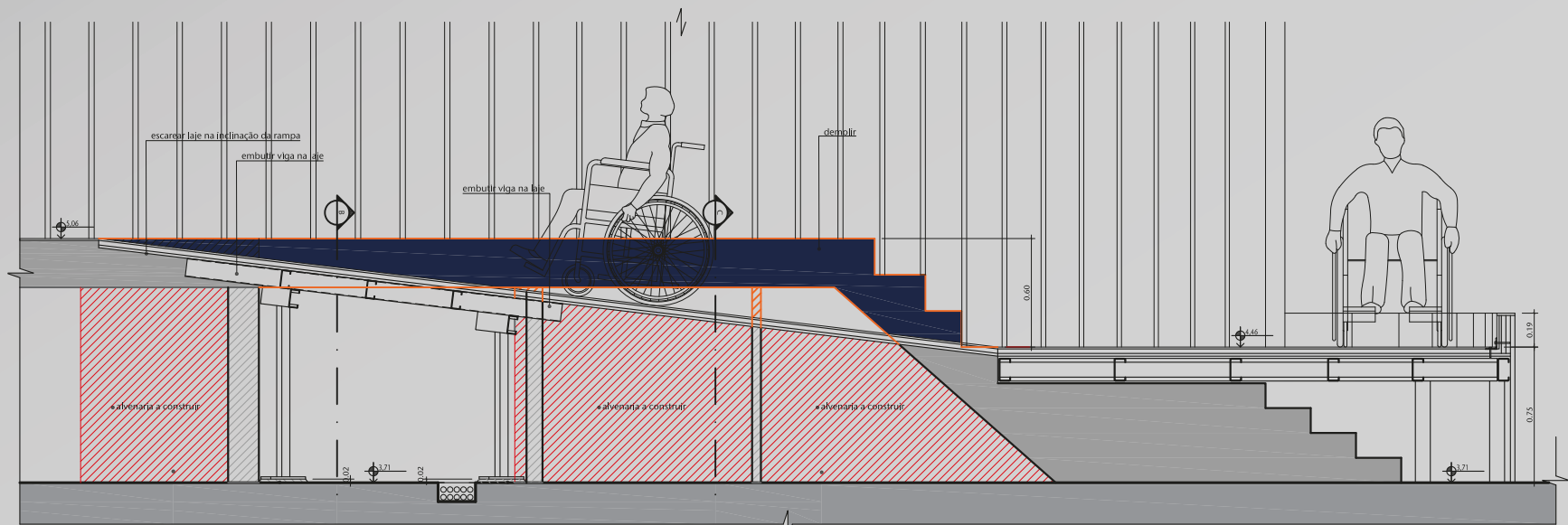
Corte transversal de la estructura de accesibilidad para la Mesa Directora del Plenario.
